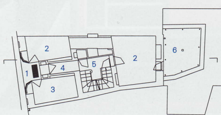
15 — Dům na Dominikánském náměstí v Brně / Půdorys 1. NP
