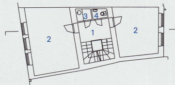
14 — Dům na Dominikánském náměstí v Brně / Půdorys 2. NP a 3. NP
