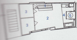
13 — Dům na Dominikánském náměstí v Brně / Půdorys mezonetu
